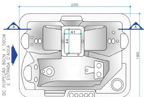
PLANTA BAIXA SPA EXTERNO ESCALA 1:25
