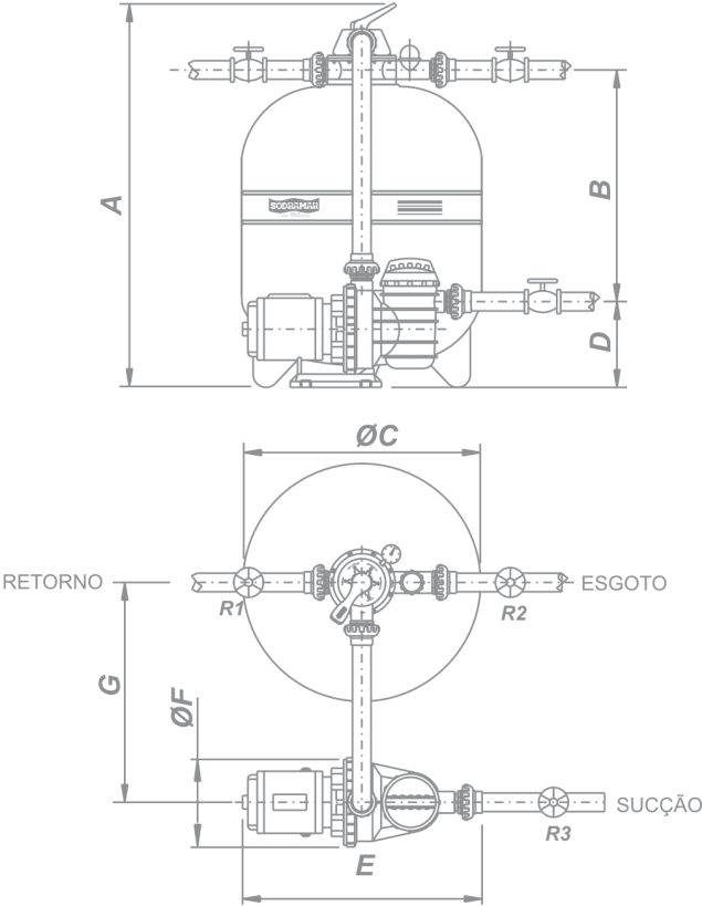
SISTEMA COM UM TANQUE F8 (INSTALAÇÃO TÍPICA)
